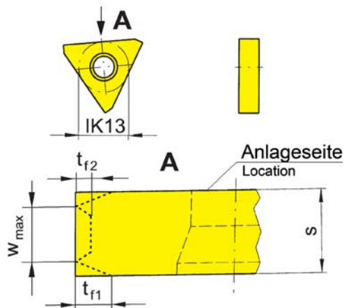
Grundabmessungen Typ 315 Basic sizes type 315
